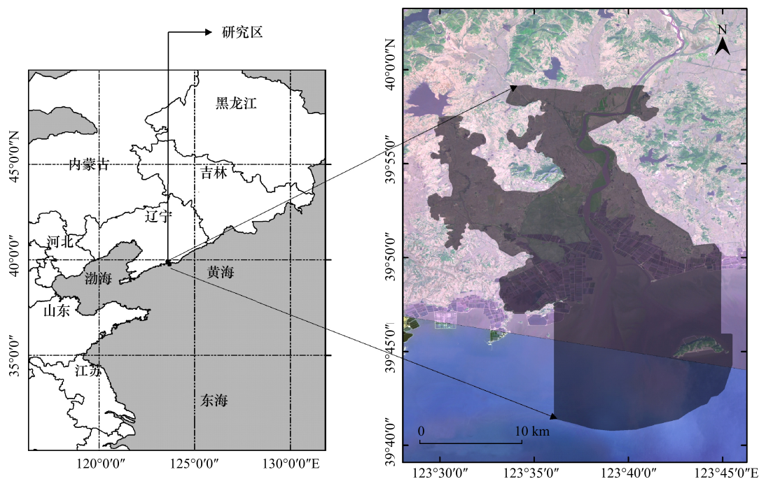
图 1 大洋河河口 2008 年 spot5 影像及位置图
