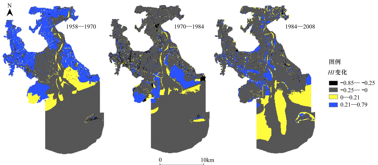
图4 不同时期人为干扰度动态度 Fig. 4 Dynamic changes of Hemeroby (HI) index at different period
