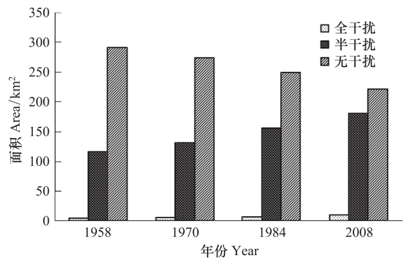
图3 人为干扰度(HI)不同干扰类型面积历史时期统计 Fig. 3 Area of different Hemeroby (HI) types at different years
