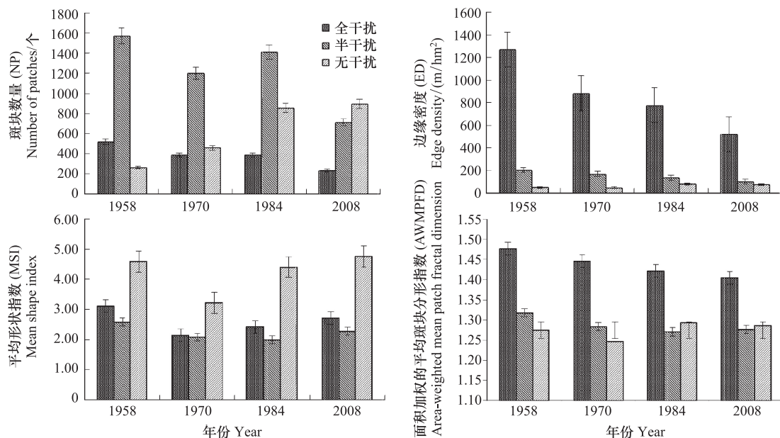
图6 不同人为干扰度景观格局指数年际变化统计
