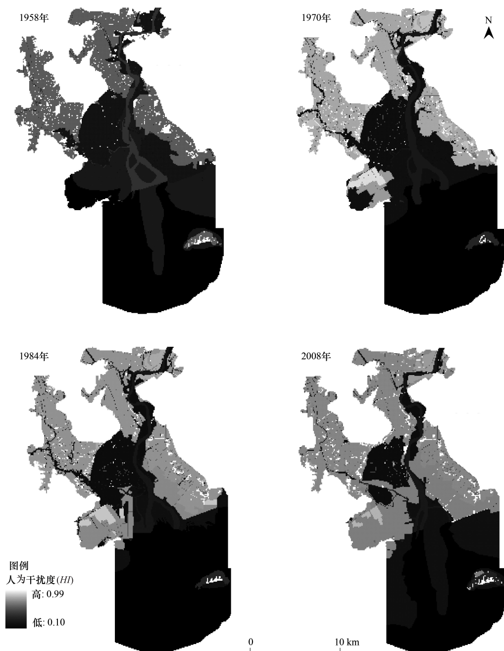
图2 不同年份大洋河河口人为干扰度(HI)
