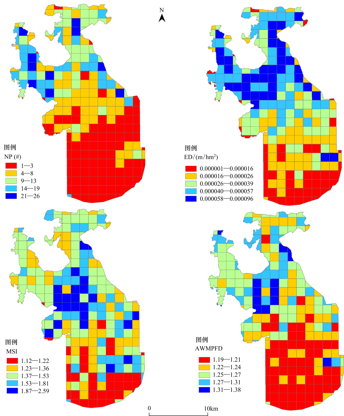
图7 大洋河河口 2008 年景观格局指数空间分异
