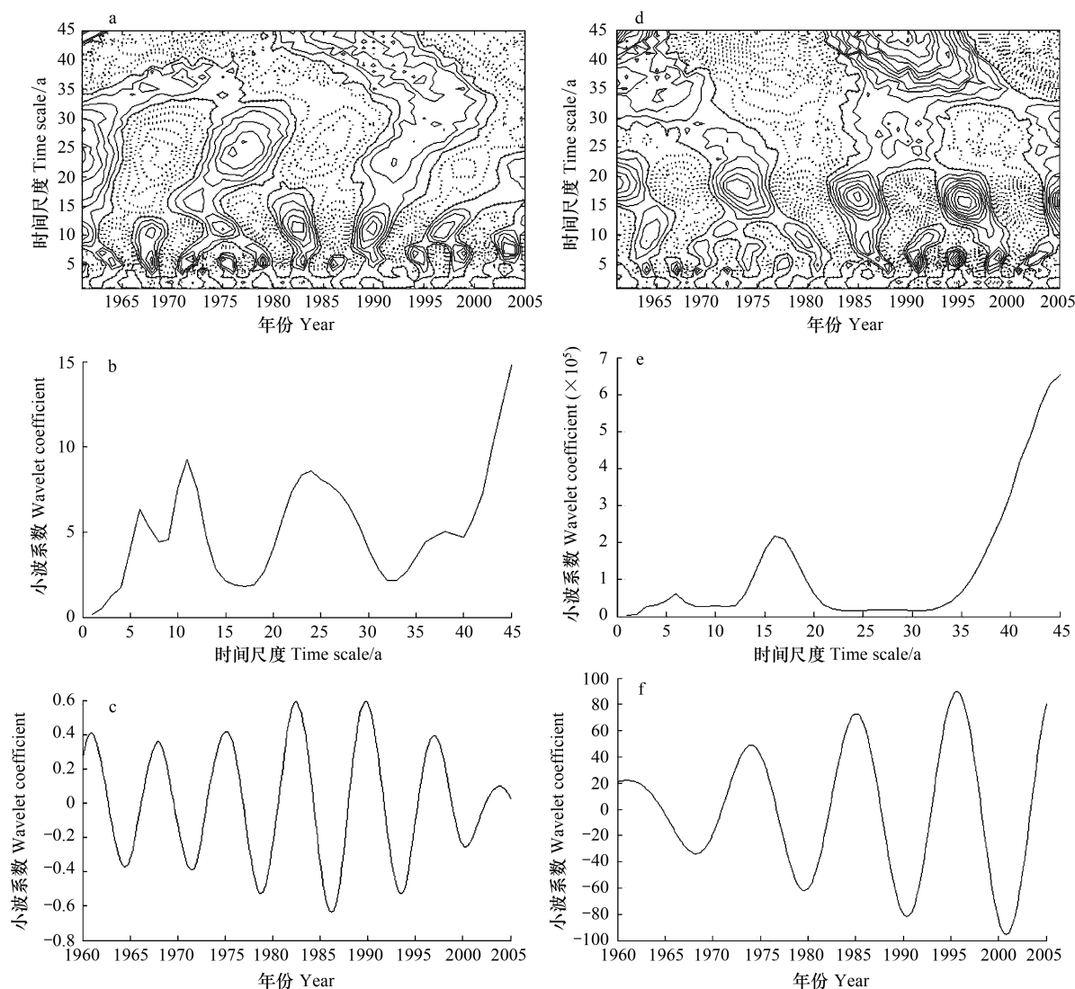
图 8 小波变换系数实部等值线图、小波方差图、主周期小波系数过程线
