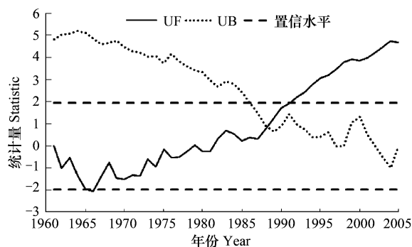
图 4 东北地区年平均气温 Mann-Kendall 突变判别曲线
