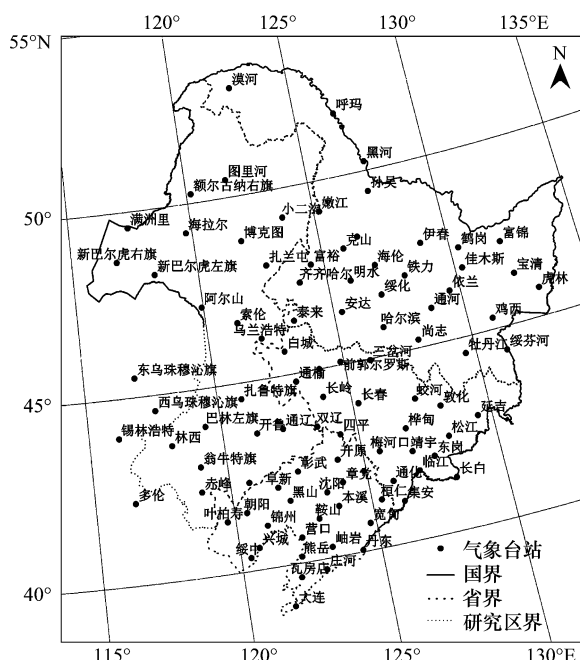
图 1 东北地区 96 个气象站点分布图
