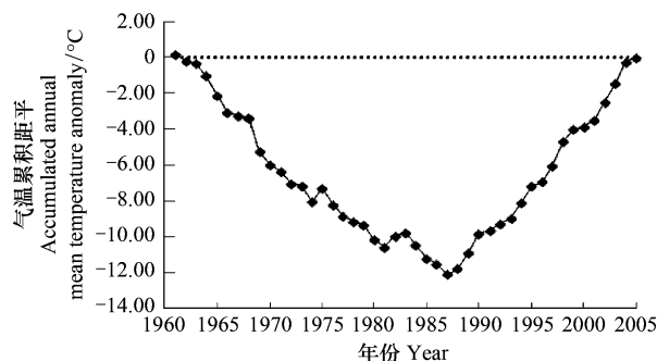
图 5 东北地区年平均气温累积距平值
