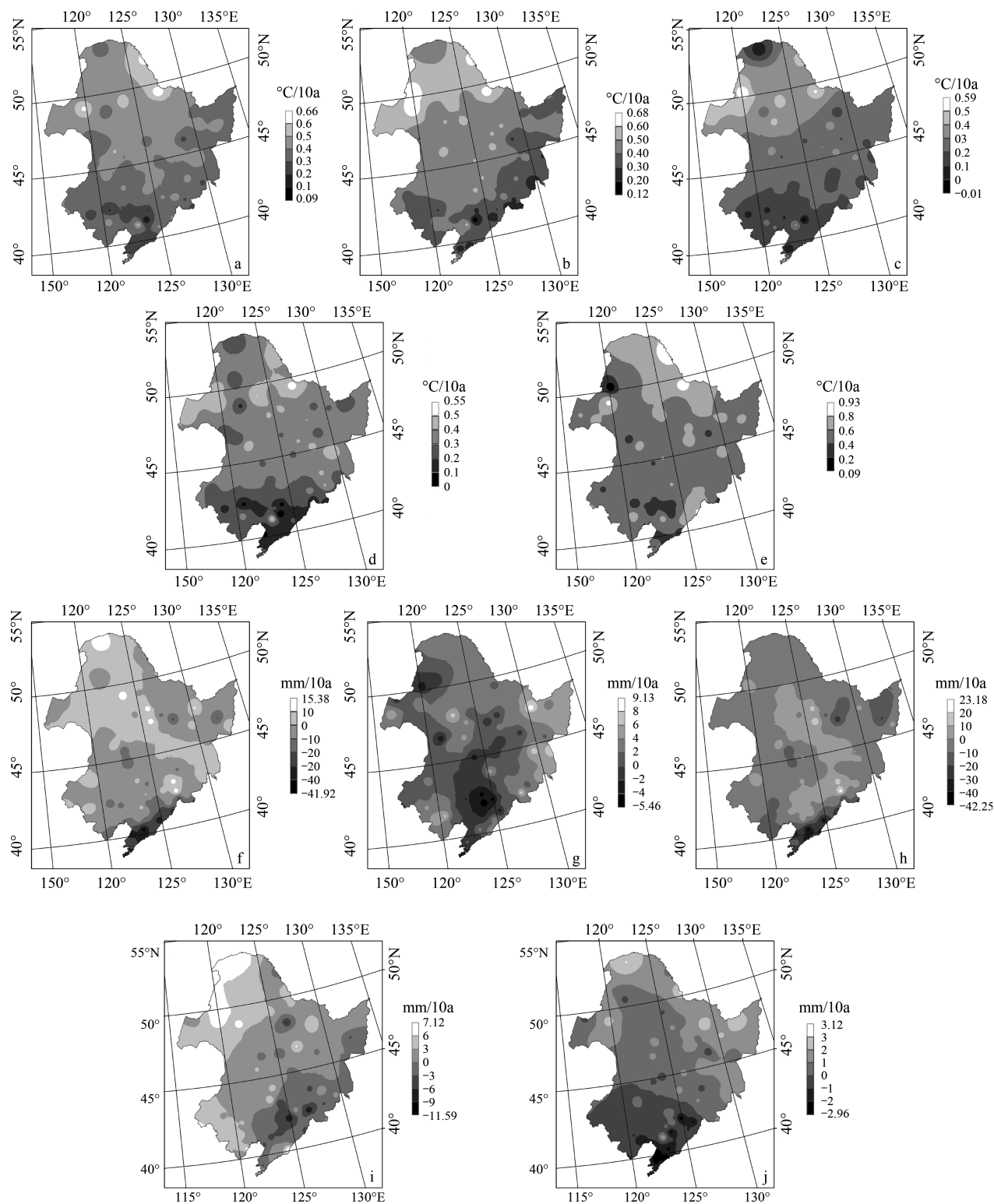
图3 东北地区气温与降水量变化趋势分布
