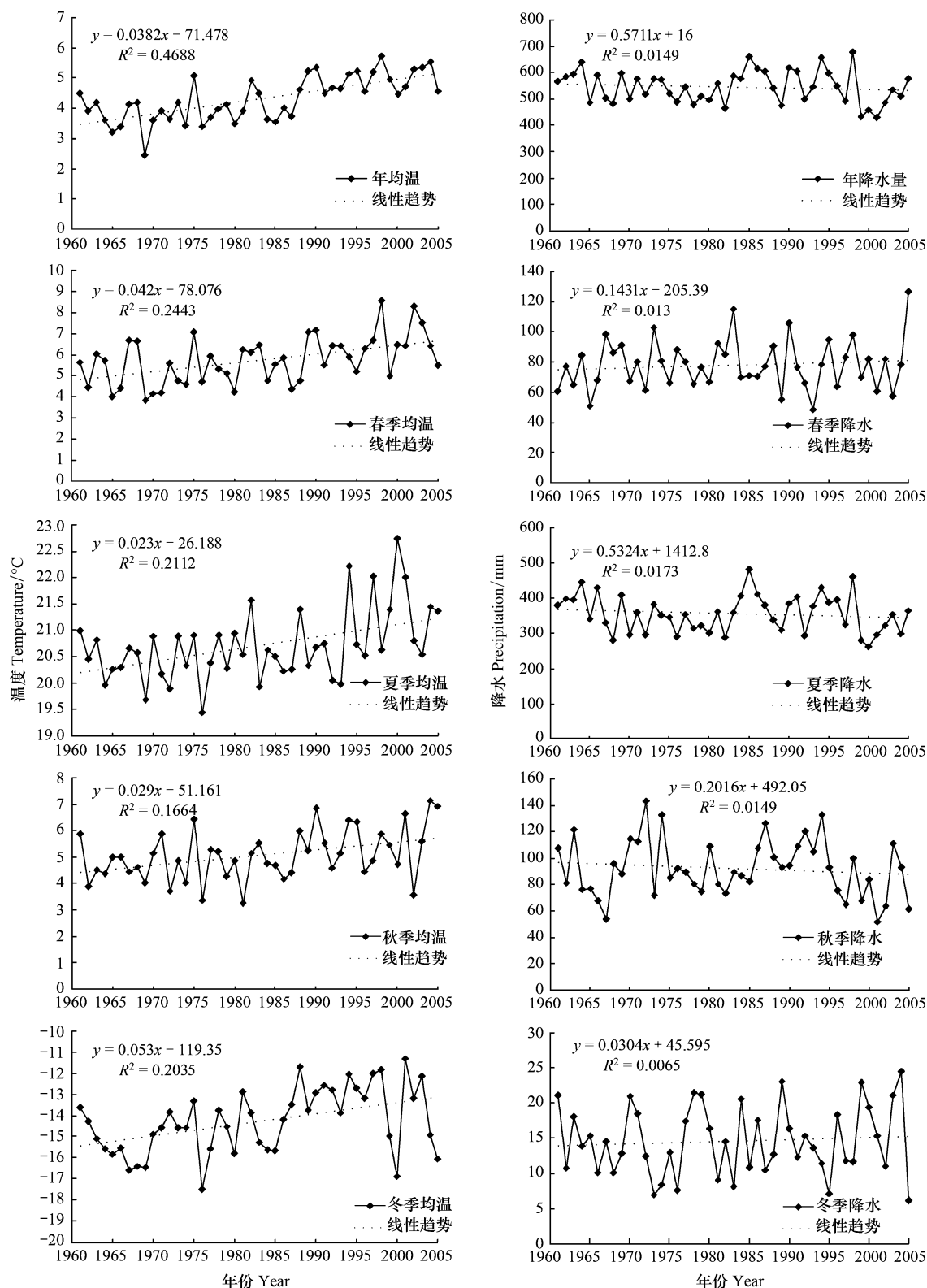
图 2 东北地区气温与降水量的年、季节变化图
