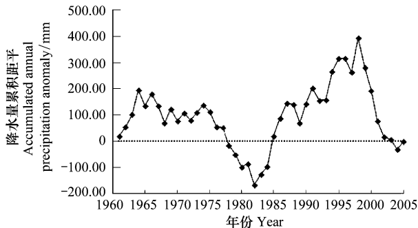
图 7 东北地区年降水量累积距平值
