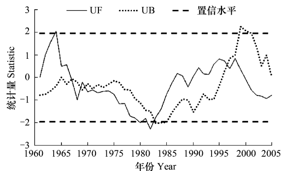
图 6 东北地区年降水量 Mann-Kendall 突变判别曲线
