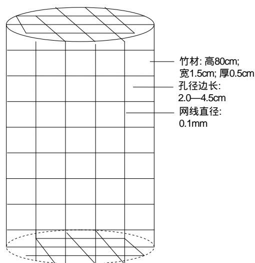
图 1 圆柱体虫网诱捕器结构图
