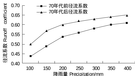
图 1 北京城区暴雨径流系数 70 年代前后变化对比 [21]
