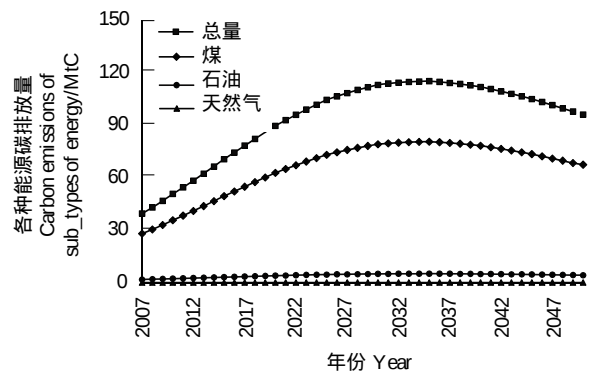
图 3 2007—2050 年各种能源碳排放预测趋势图
