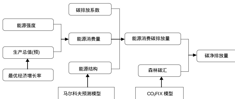
图1 云南省碳净排放计算流程图
