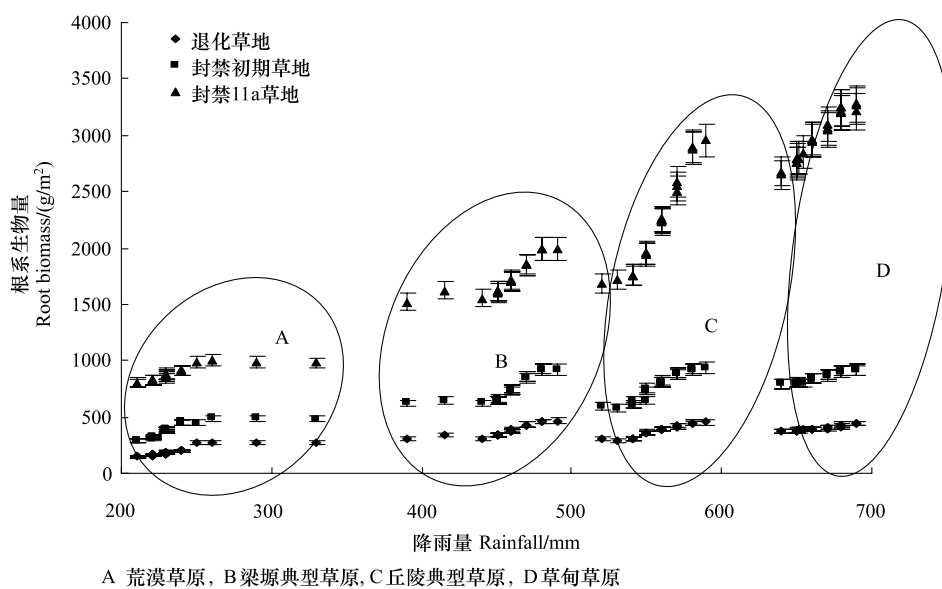
图 3 草地 0—100cm 根系生物量与降雨量空间分布
