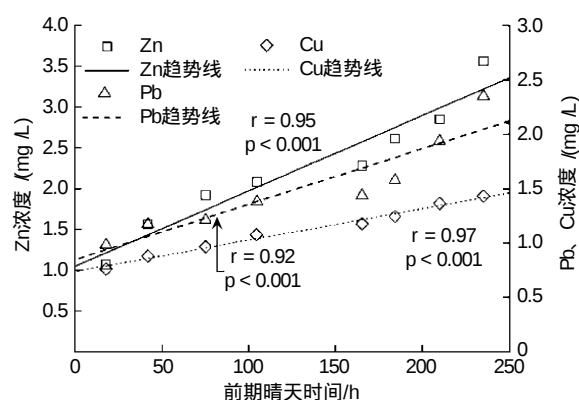
图 2 地表径流中重金属浓度与前期晴天时间的关系 [74]
