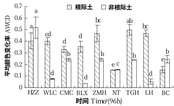
图2 不同植物土壤微生物 AWCD(96h)比较 Fig. 2 Average well color development under different species of plant 图中小写字母(a,b,c,d和e)表示不同植物类型间在0.05水平上的差异
