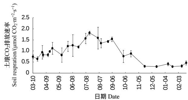
图2 裸地土壤呼吸速率的季节变化
