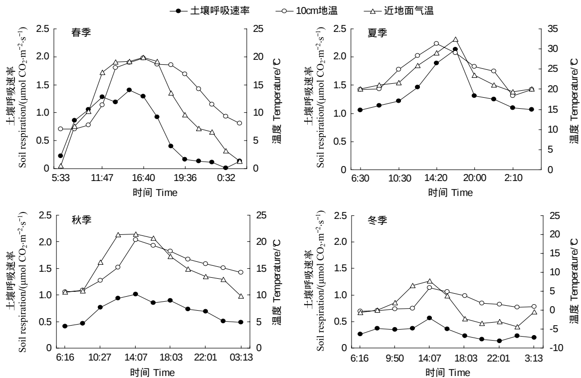
图1 裸地土壤呼吸速率日变化
