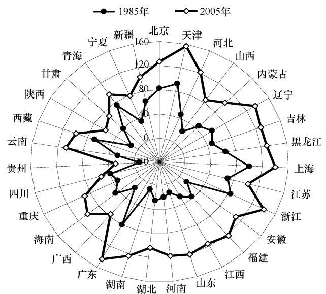
图 1 1985—2005 年中国各省份土地利用总功能变化
