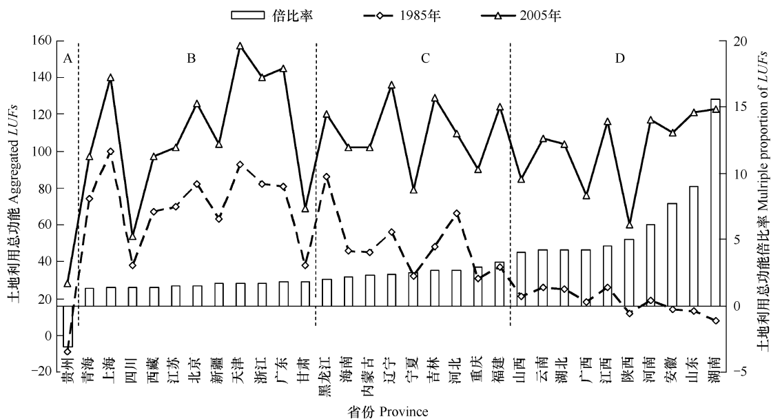
图 2 1985—2005 年中国各省份土地利用功能变化倍比率
