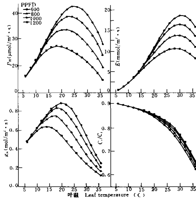
图1 用光合作用-蒸腾作用-气孔导度的耦合模型模拟的生理因子随叶温的变化
