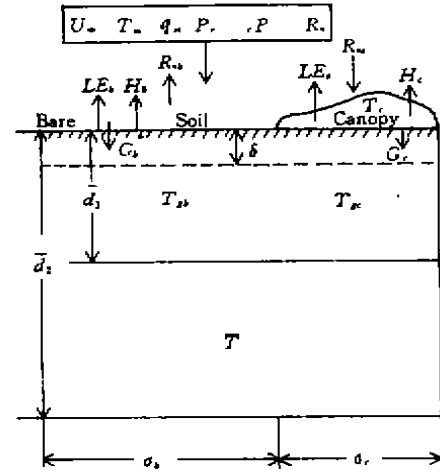
图 2 地表热量输出示意图
