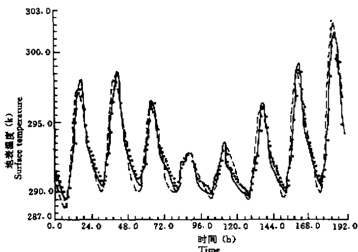
图3 地表温度随时间的变化
