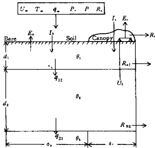
图 1 水分运动示意图
