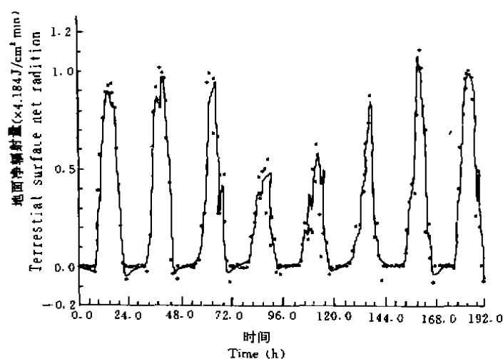
图6 地面净辐射量随时间的变化
