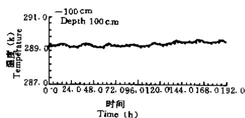
图 4 100cm 深处土壤温度随时间的变化
