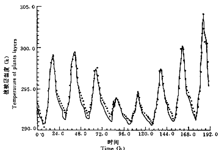
图 5 植被层温度随时间的变化
