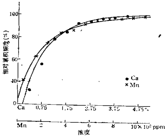
图1 Ca和Mn的分布概率曲线图
