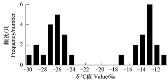
图2 越冬代棉铃虫雌蛾翅稳定同位素碳比值分布图
