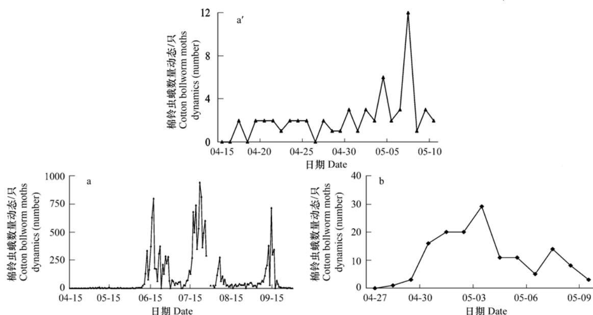
图 1 2007 年黑光灯上棉铃虫蛾(a)和越冬代春季羽化棉铃虫数量动态(a')及 2007 年杨树把诱集越冬代棉铃虫春季羽化数量动态(b)
