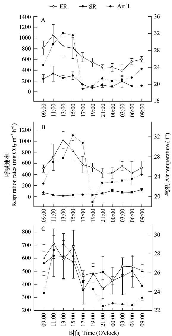
图 1 生态系统呼吸、土壤呼吸和大气温度在拔节期(A)、抽穗开花期(B)和收割后 3d(C)的日变化
