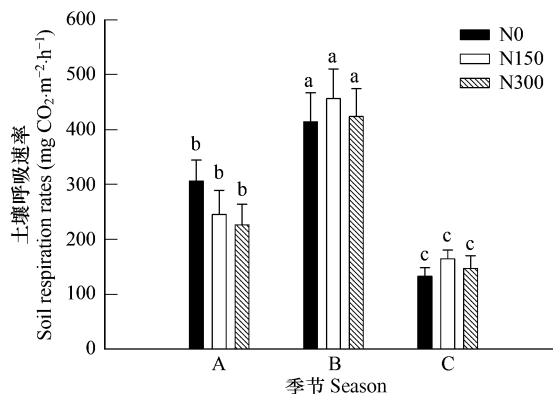
图2 不同季节不同氮肥水平土壤呼吸速率平均值
