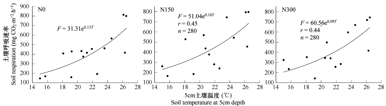
图4 水稻收割后氮肥水平处理土壤呼吸与土壤温度的关系
