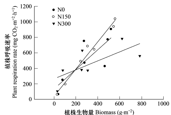
图5 不同氮肥水平处理植株呼吸与植株生物量的关系
