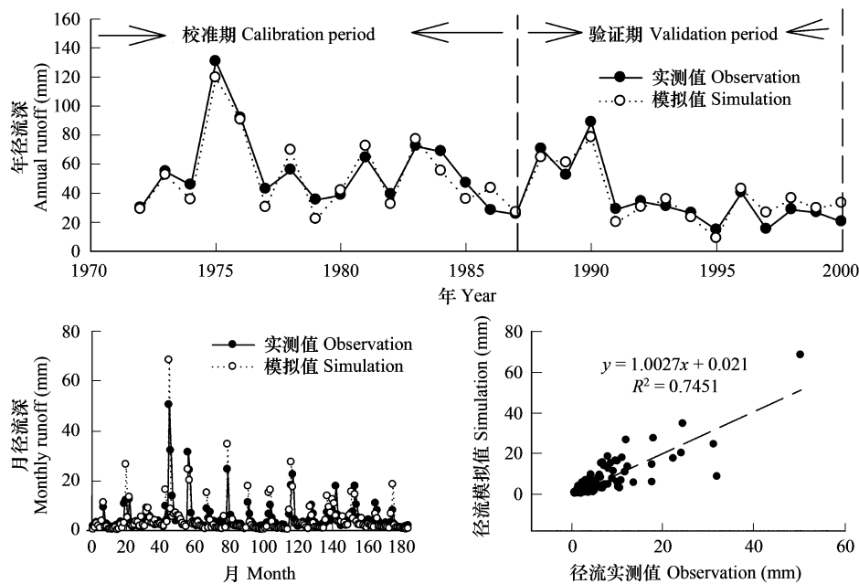
图 2 黑河流域径流量的实测值与模拟值
