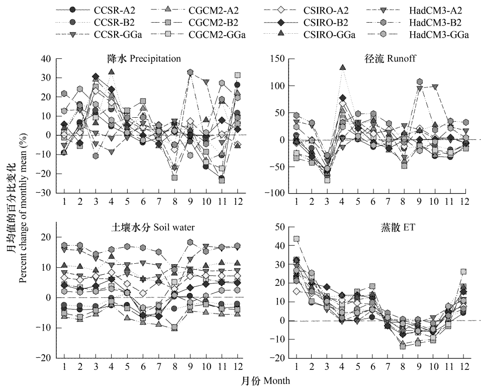
图3 2010~2039年黑河流域月均降水、径流、土壤水分和蒸散的相对变化(%)
