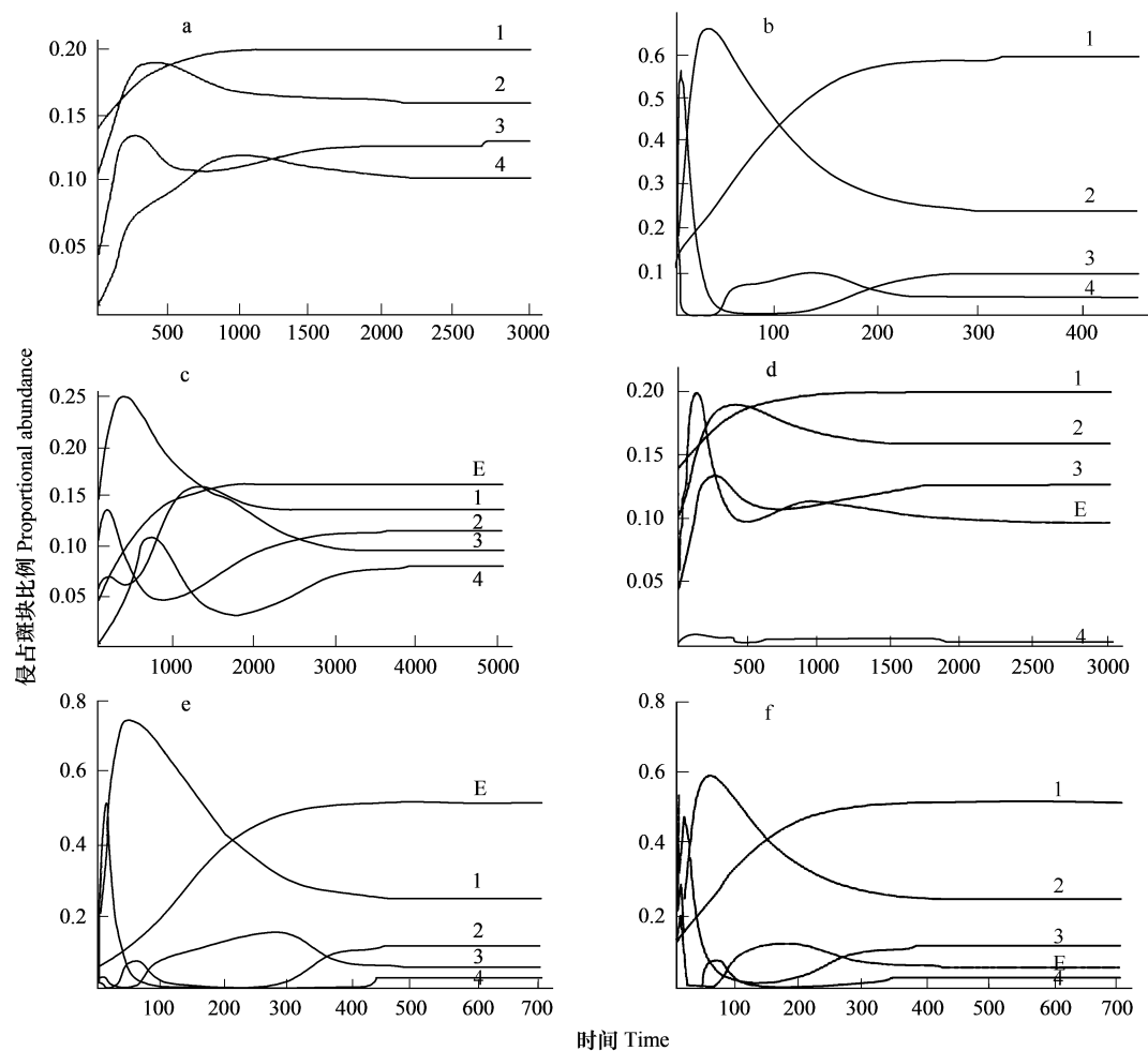
图2 外来物种入侵前后集合群落的系统动力模拟
