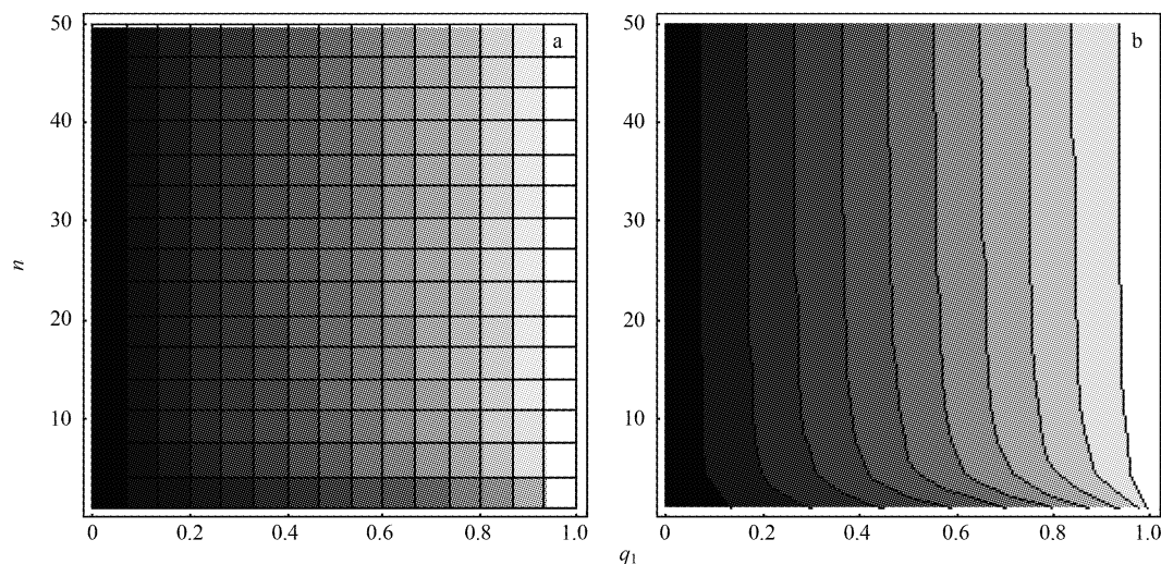
图 1 外来物种入侵后混合物种竞争力最强物种的比例稳定值 q_2 分析图
