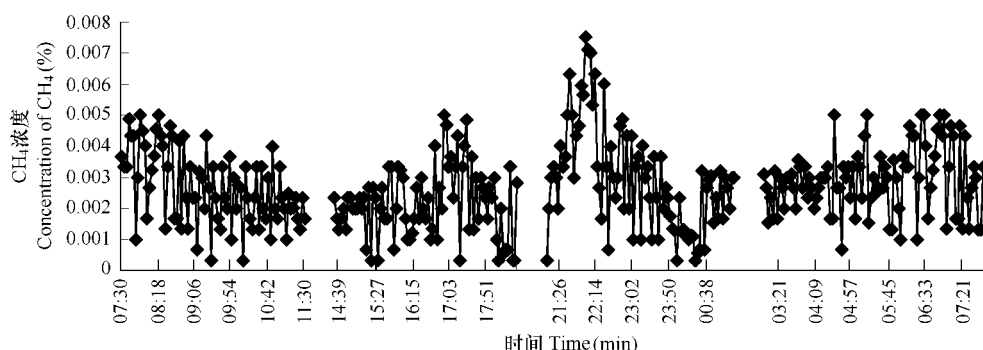
图 1 24h 内不同时间点箱内 \text{CH}_4 浓度
