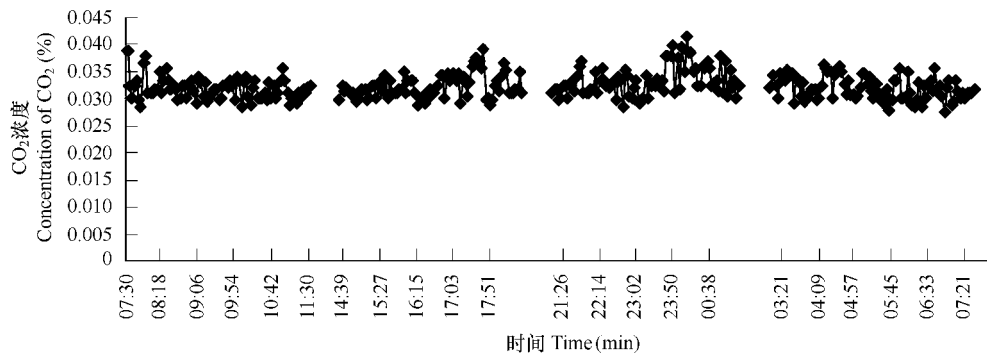
图2 24h内不同时间点箱内CO 2 浓度
