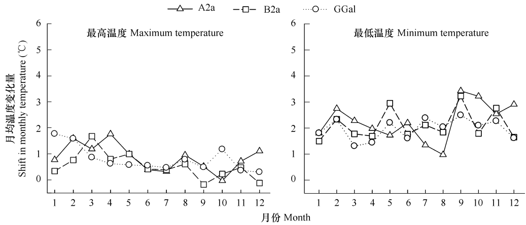
图3 3种情景预测的2010~2039年相较于1957~2001年的最高、最低温度的变化
