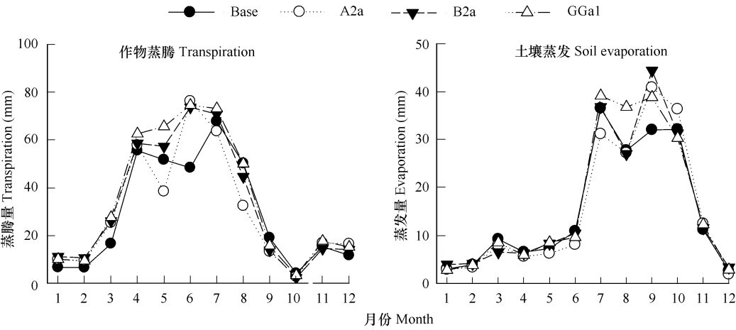
图4 作物蒸腾与土壤蒸发的月变化
