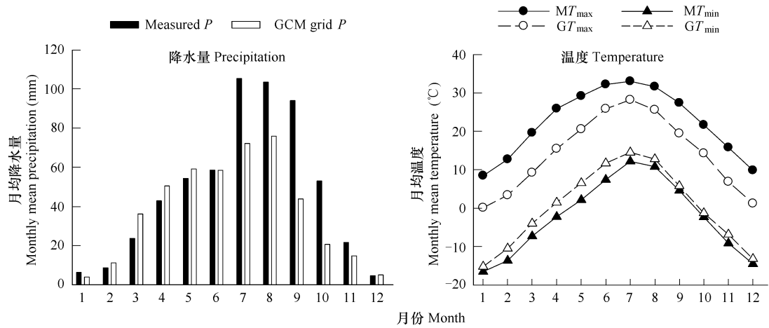
图 1 1957 ~ 2001 年 GCM 网格的与实测的月降水量、最高和最低温度的差异
