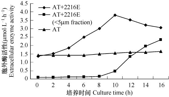
图4 溶藻过程中氨肽酶活性变化
