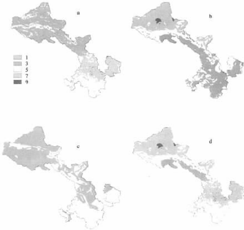
图 1 甘肃省生态环境敏感性分布图
