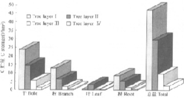
图 2 各亚层干、枝、叶、根的 C 贮量
