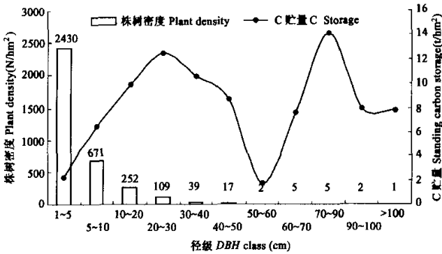
图 1 C 贮量和株数密度的径级分布
