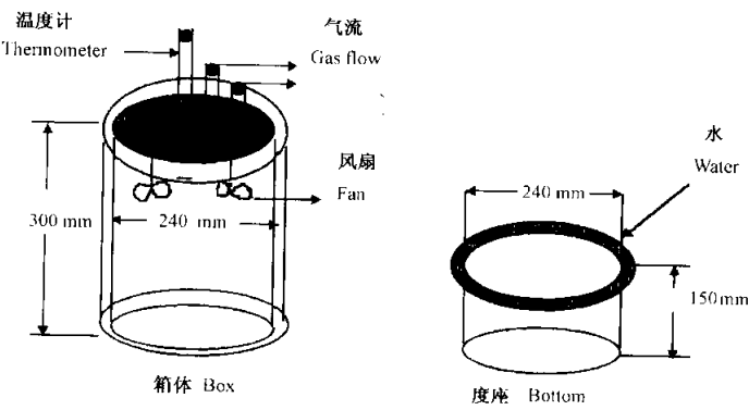
图 1 气体采集箱 Fig. 1 Gas collected box
